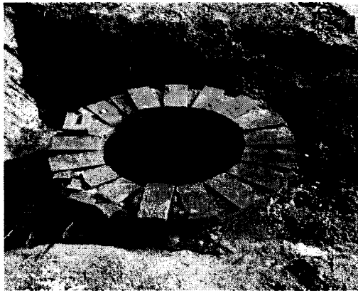
CONSTRUCCION DE POZO DE VISITA LISTO PARA RECIBIR BROCAL Y TAPA
